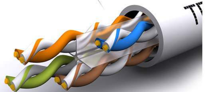
cable UTP categoría 6 rígido
