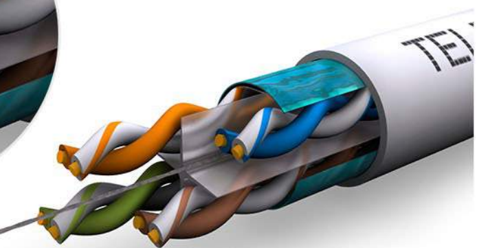
cable FTP categoría 6 rígido
