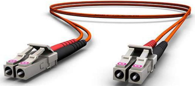
OM1 (62,5/125)
